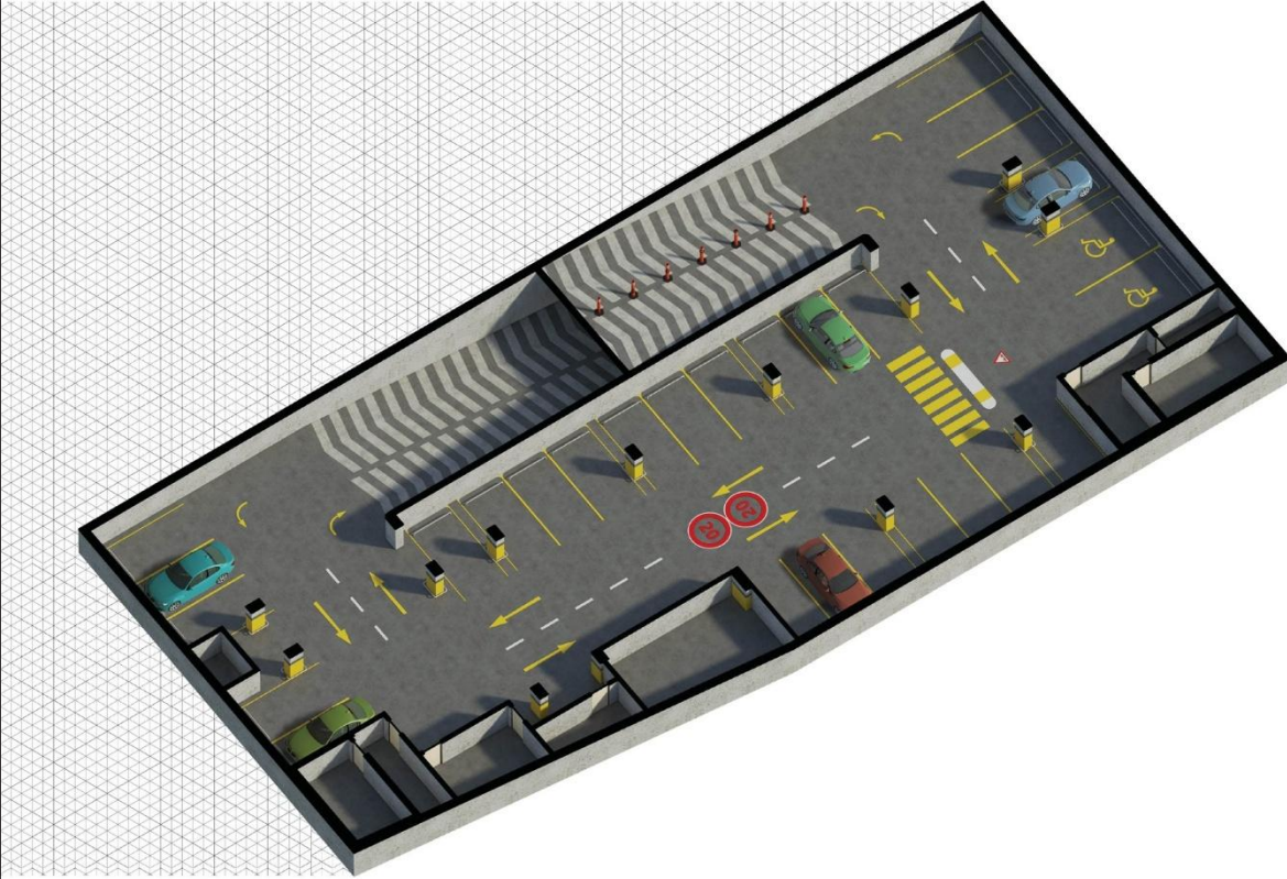
BAĞCILAR ÇOLAKOĞLU SOKAK ZEMİNALTI OTOPARK PROJESİ (BAG-23) Aksonometrik Perspektif - 2. Bodrum Katı
